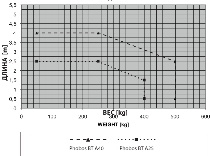
МАКСИМАЛЬНАЯ ДЛИНА/ВЕС СТОРКИ
